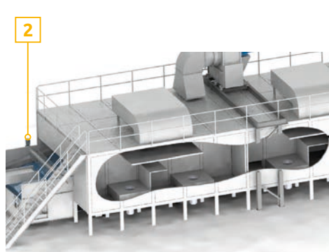
TopDown-Kammer Luftrichtung durch das Band von unten nach oben
